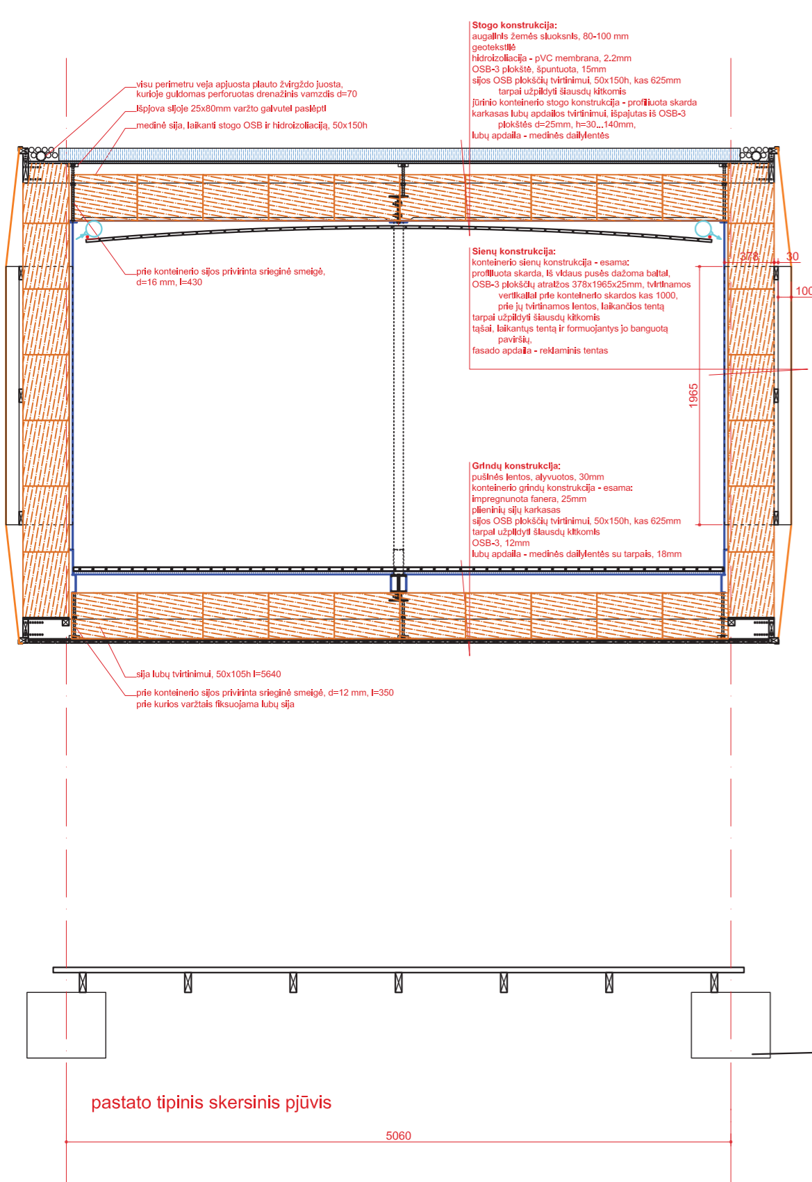
pastato skersinis pjūvis
